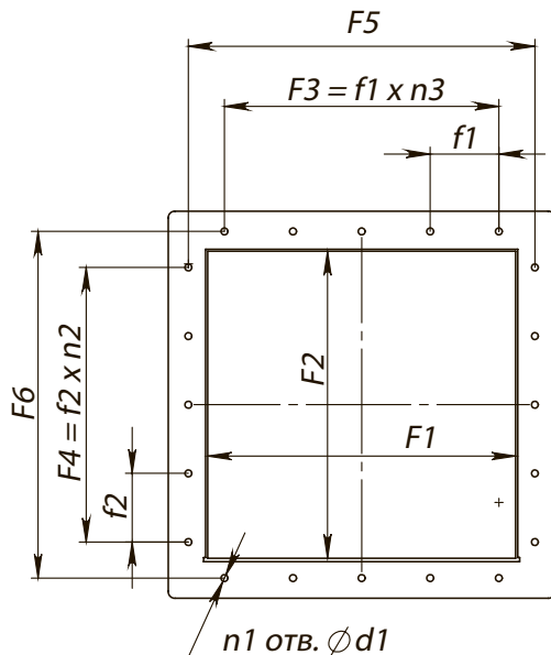
Вид Е
