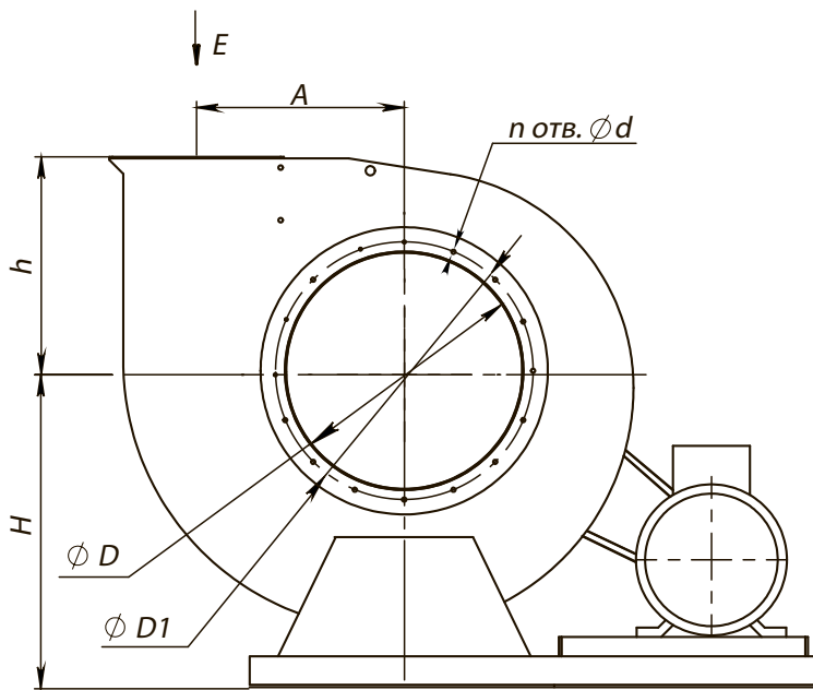
Вид Е
