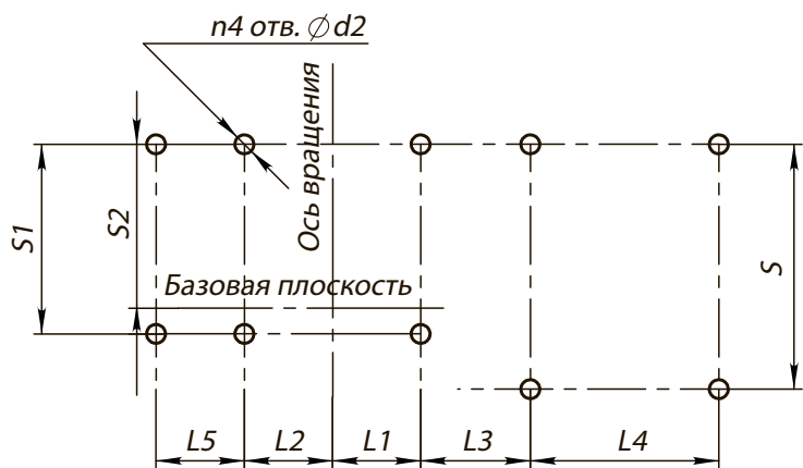
Схема расположения отверстий для крепления вентилятора
