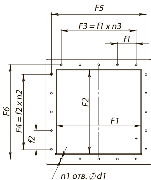
Вид Е
